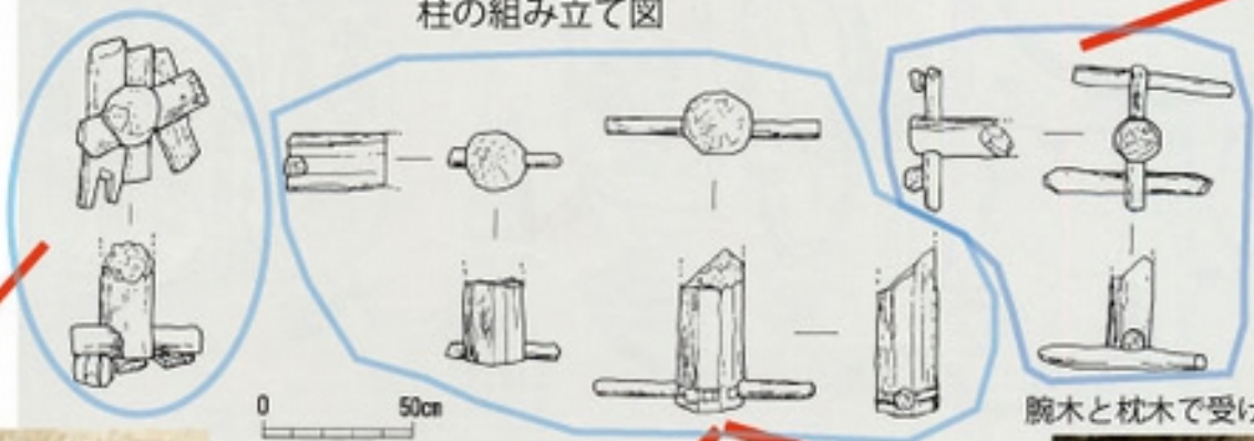
柱の組み立て図
