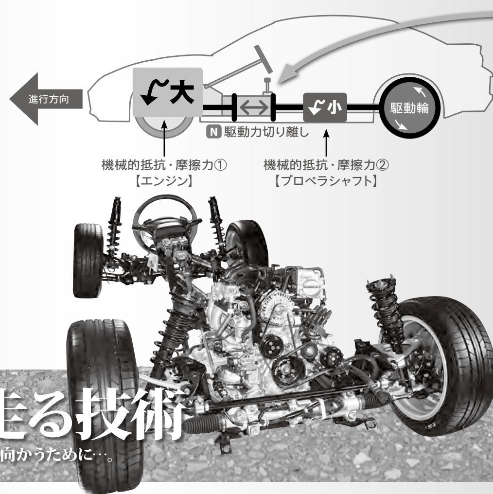
エンジンとオートマチックトランスミッション
