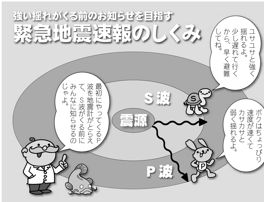
P波(初期微動): 秒速約7km S波(おもに被害をもたらす主要動): 秒速約4km
